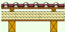
LINITHERM PAL N+F na dřevěné bednění
